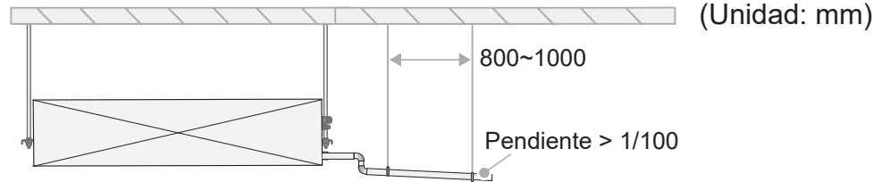
Método para conectar la tubería de drenaje para una unidad simple
