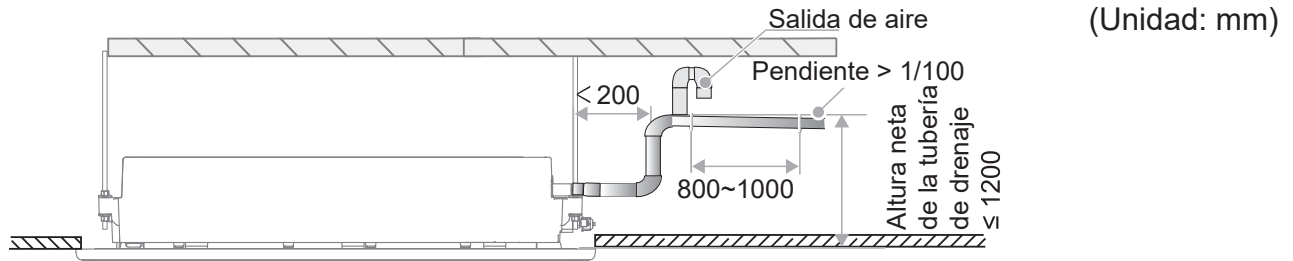
Cómo conectar la tubería de drenaje para la bomba de drenaje de una unidad simple
